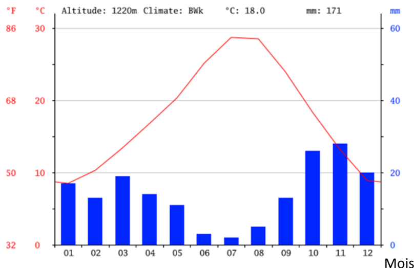
Figure 2 : Diagramme ombro-thermique pour Skoura (source : climate-data.org, 2015)
